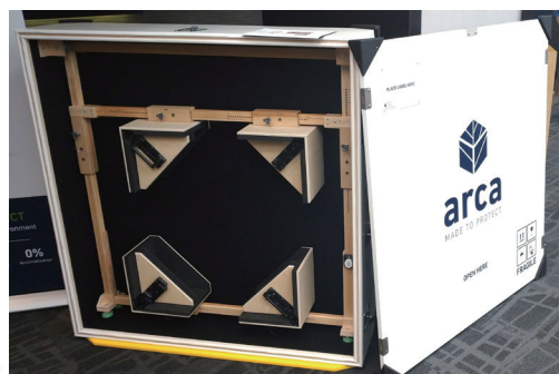
図8-2 内部構造
