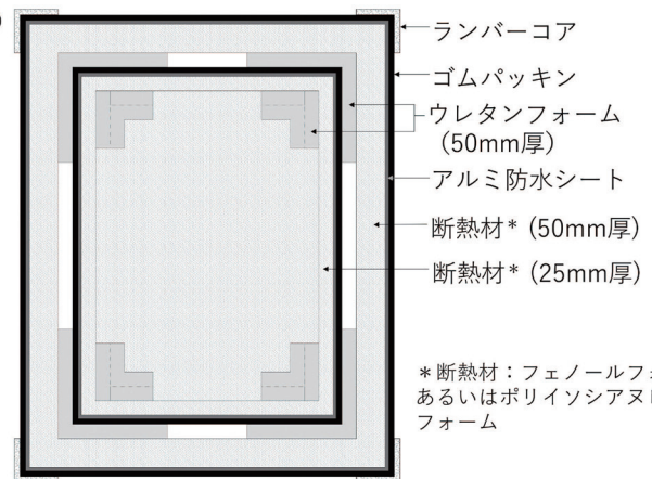
図1 西美の使い捨てクレート（二重箱）の構造（上：断面図、右：平面図）。作品は薄葉紙でくるんだあとポリエチレンシートで包み、ビニールテープで密閉して内箱に取める。ウレタンフォーム（スポンジ）は、作品の重量や額の形状にあわせて、都度、適切な固さのものを選択する。箱躯体と蓋が密閉するように、本体と蓋が合わさる箇所にはゴムパッキンを回してある。外箱は防水のために塗装するが、内箱は塗装しない。一重箱の場合は、この図で示した内箱のみの構造となり、箱に塗装は行わない。
