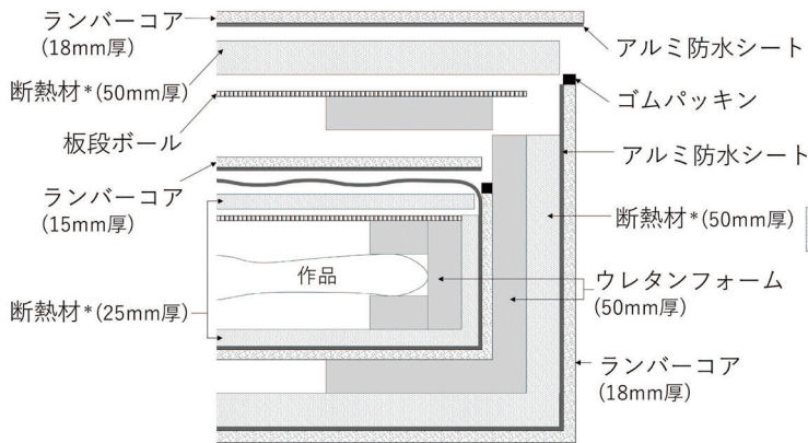
図1 西美の使い捨てクレート（二重箱）の構造（上：断面図、右：平面図）。作品は薄葉紙でくるんだあとポリエチレンシートで包み、ビニールテープで密閉して内箱に取める。ウレタンフォーム（スポンジ）は、作品の重量や額の形状にあわせて、都度、適切な固さのものを選択する。箱躯体と蓋が密閉するように、本体と蓋が合わさる箇所にはゴムパッキンを回してある。外箱は防水のために塗装するが、内箱は塗装しない。一重箱の場合は、この図で示した内箱のみの構造となり、箱に塗装は行わない。
