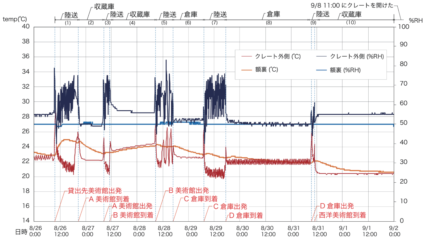
図3 西美からライクスミュージアムへの輸送時における温度・湿度変化。輸送過程:クレートを美術品輸送専門車によって成田空港まで運び(グラフ上部のバーの(1))、旅客機に搭載して(2)、輸送した(3)。スキポール空港到着後、旅客機から荷下ろしし(4)、美術品輸送専門車に積みなおしてライクスミュージアムまで運び(5)、収蔵庫で保管(6)。シーズニング後、開梱。
